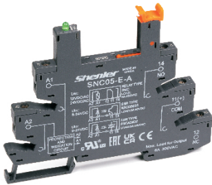
插座
