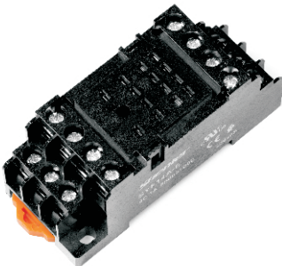
插座
