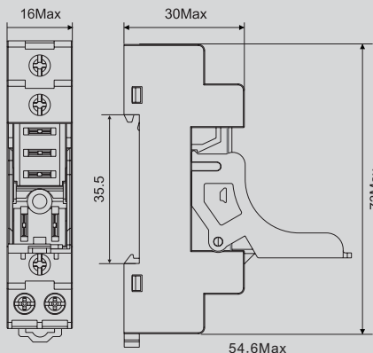
SRT05-ES
