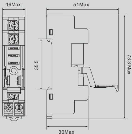
SRT05-ES
