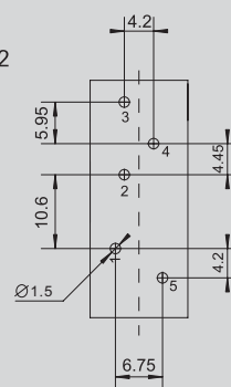
SRT05-P 底视图
